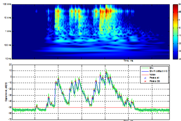
Частотно-временная характеристика контактора РПН (источник: A2-204, K. Viereck, A. Saveliev, U. Sundermann , M. Späth )
