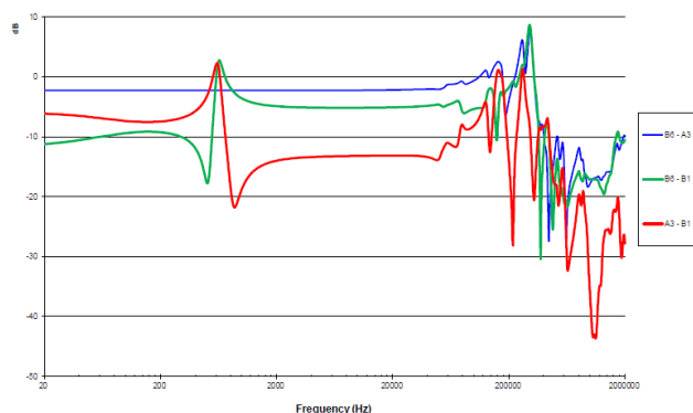
Передаточные функции напряжения на регулировочных выводах обмотки (источник: A2-215, J.A. Lapworth, P.N. Jarman, Z.D. Wang and S. Dragostinov)
